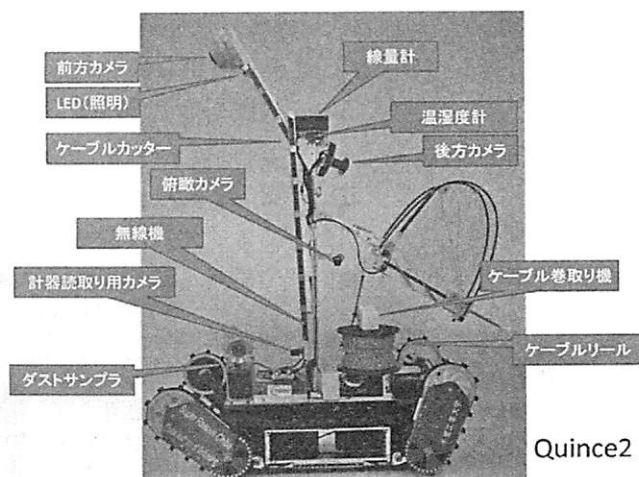
写真—1 福島第一原子力発電所の原子炉建屋内調査に導入された Quince（千葉工大 小柳栄次氏提供）
