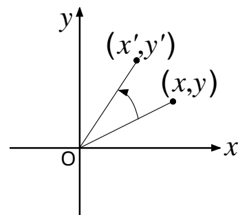
図 2 点の回転
