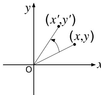
図2 点の回転
